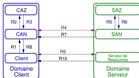
FIGURE 5.1 – Modèle de l'architecture ACE DCAF.
