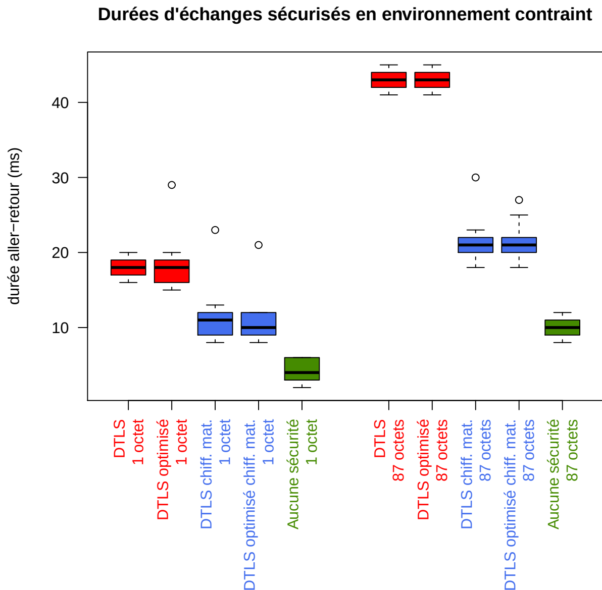
FIGURE 7.4 – Aller-retour de messages, avec un seul octet puis 87 : DTLS, DTLS optimisé, leur variante avec chiffrement matériel et enfin sans DTLS.
