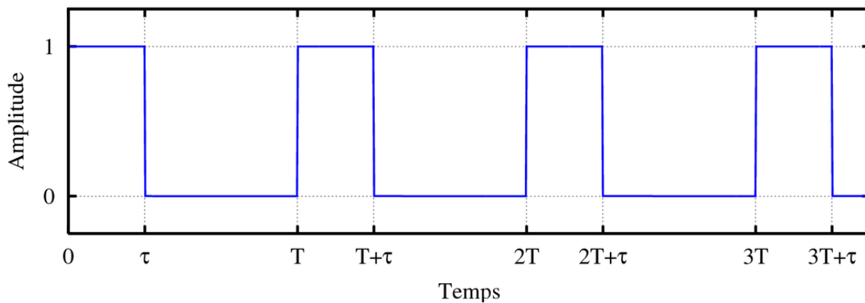
FIGURE 2.2 – Fonctionnement du rapport cyclique. Pour une radio, nous pouvons considérer l'amplitude de 1 comme une radio activée, 0 comme une radio éteinte. Le rapport cyclique est ici de \frac{\tau}{T} , avec \tau l'intervalle de temps pendant laquelle la radio est activée et T la période. (extrait de Wikipédia)
